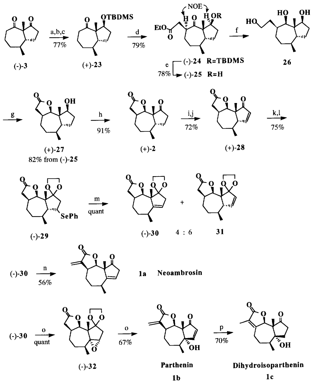
Scheme 5. a) DIBAH, THF, -78 °C; b) TBDMSCl, imidazole, DMF, 0 °C; c) PDC, CH 2 Cl 2 , π; d) LDA, ICH 2 CO 2 Et, HMPA, THF, -78 °C; e) AcOH-H 2 O-THF, 100 °C; f) DIBAH, THF; g) PtO 2 , O 2 ; h) Jones ox.; i) TMSOTf, Et 3 N; j) Pd(OAc) 2 ; k) PhSeH, AcOH; l) (TMSOCH 2 ) 2 , TMSOTf, 0 °C; m) NaIO 4 , MeOH-H 2 O, 0 °C; n) ref. 15; o) ref. 5; p) ref. 3a.
